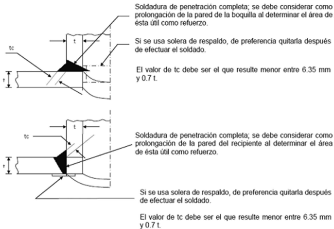
FIGURA A.2 ALGUNOS TIPOS PERMITIDOS DE BOQUILLAS SIN ESFUERZO
