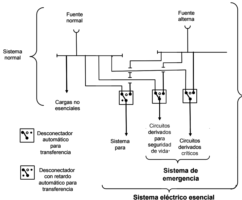
FIGURA 517-30 (a).- Hospitales y lugares de atención de la salud para pacientes ambulatorios – Requisito mínimo de desconectados para transferencia.
