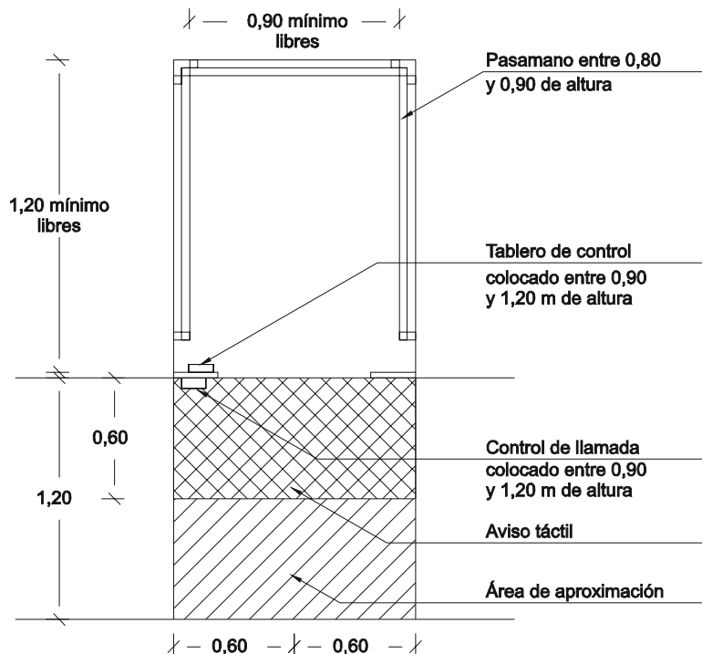
Elevador
