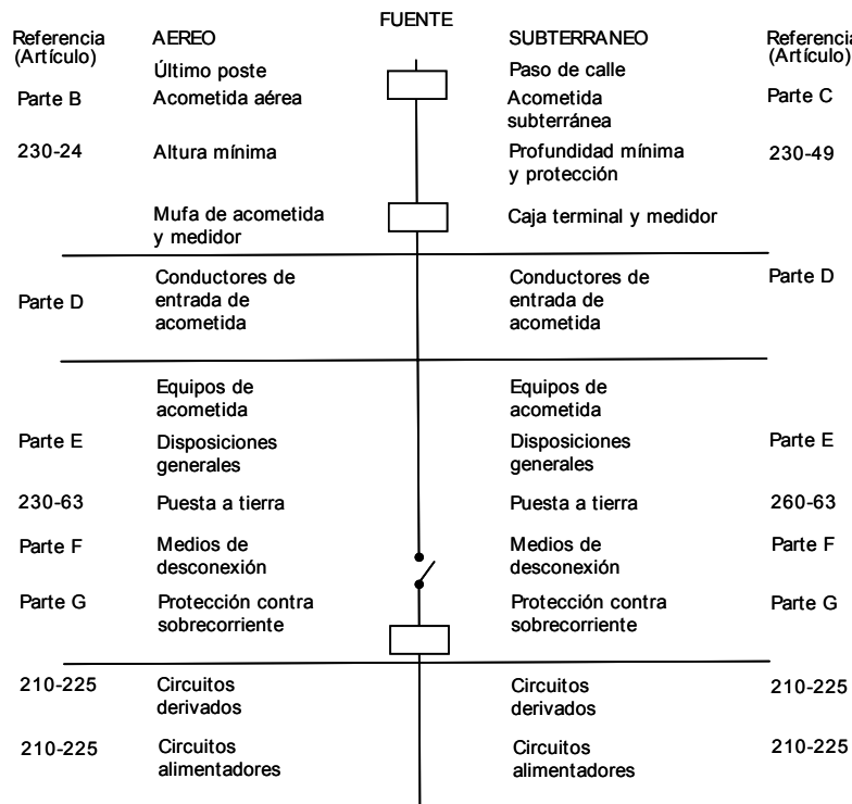
FIGURA 230-1.- Acometidas
