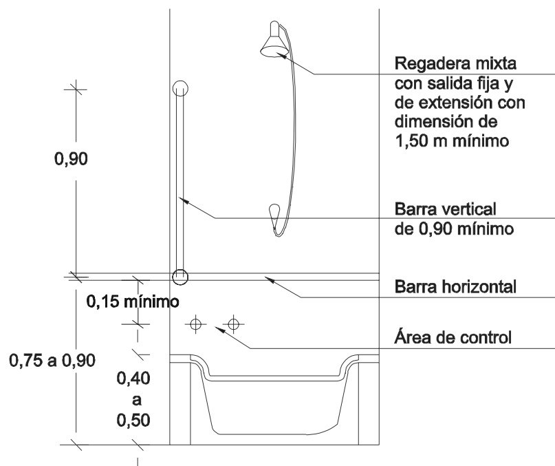
Tina alzado (vista frontal)
