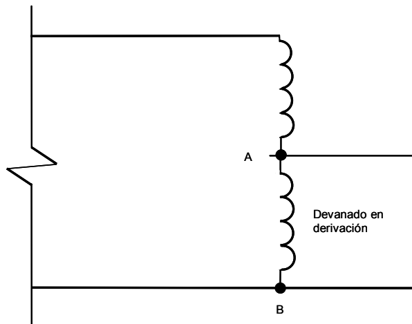
FIGURA 450-4.- Autotransformador
