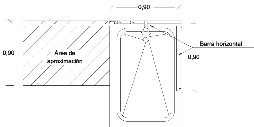
Tina (planta)
