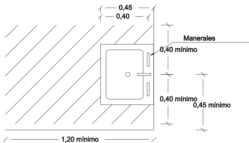
Lavamanos planta
