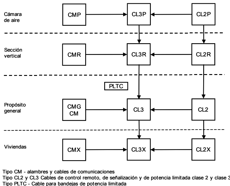
FIGURA 725-61.- Jerarquía de sustitución de los cables
