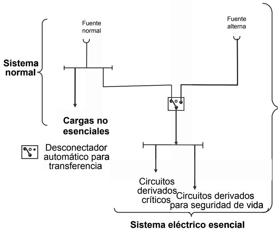
FIGURA 517-41 (b) Enfermerías y lugares de cuidados de la salud para la atención a pacientes con limitaciones – Requisito mínimo de un desconector para transferencia con carga de hasta 150 KVa.
