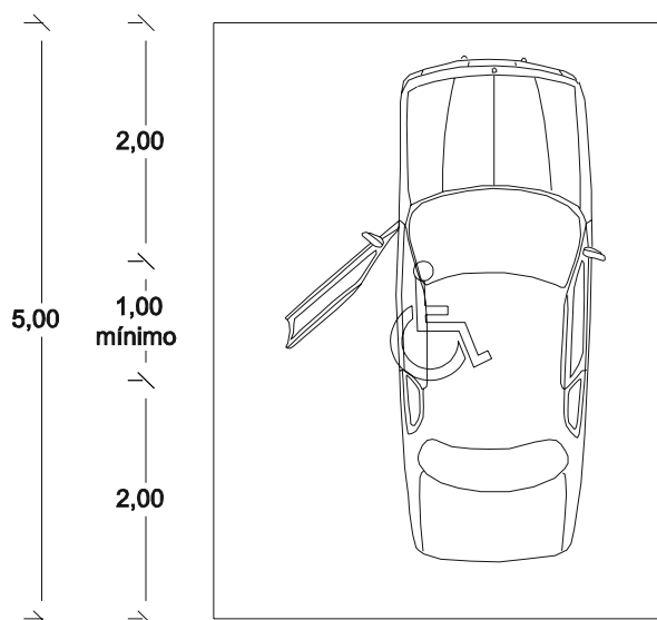
Ruta accesible
