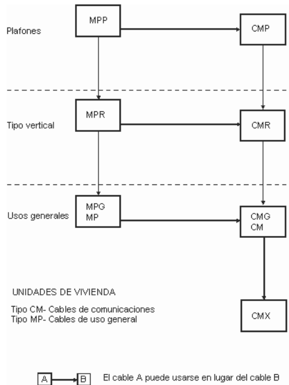
Figura 800-53.- Jerarquía de sustitución de cables
