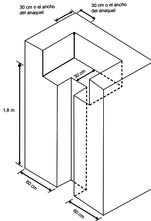
FIGURA 410-8.- Espacio de almacenamiento del clóset
