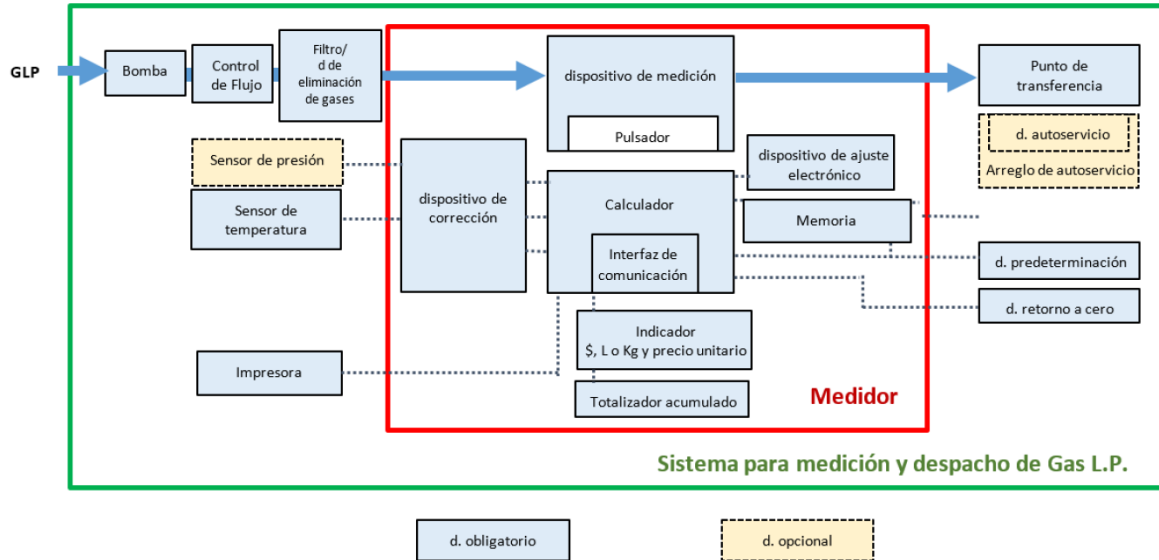
Figura Ilustrativa 1. Componentes de un Sistema para medición y despacho de Gas L.P.
