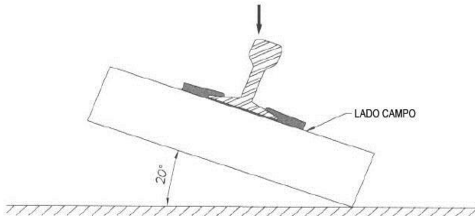
Figura 15. Prueba de carga repetitiva de la fijación
