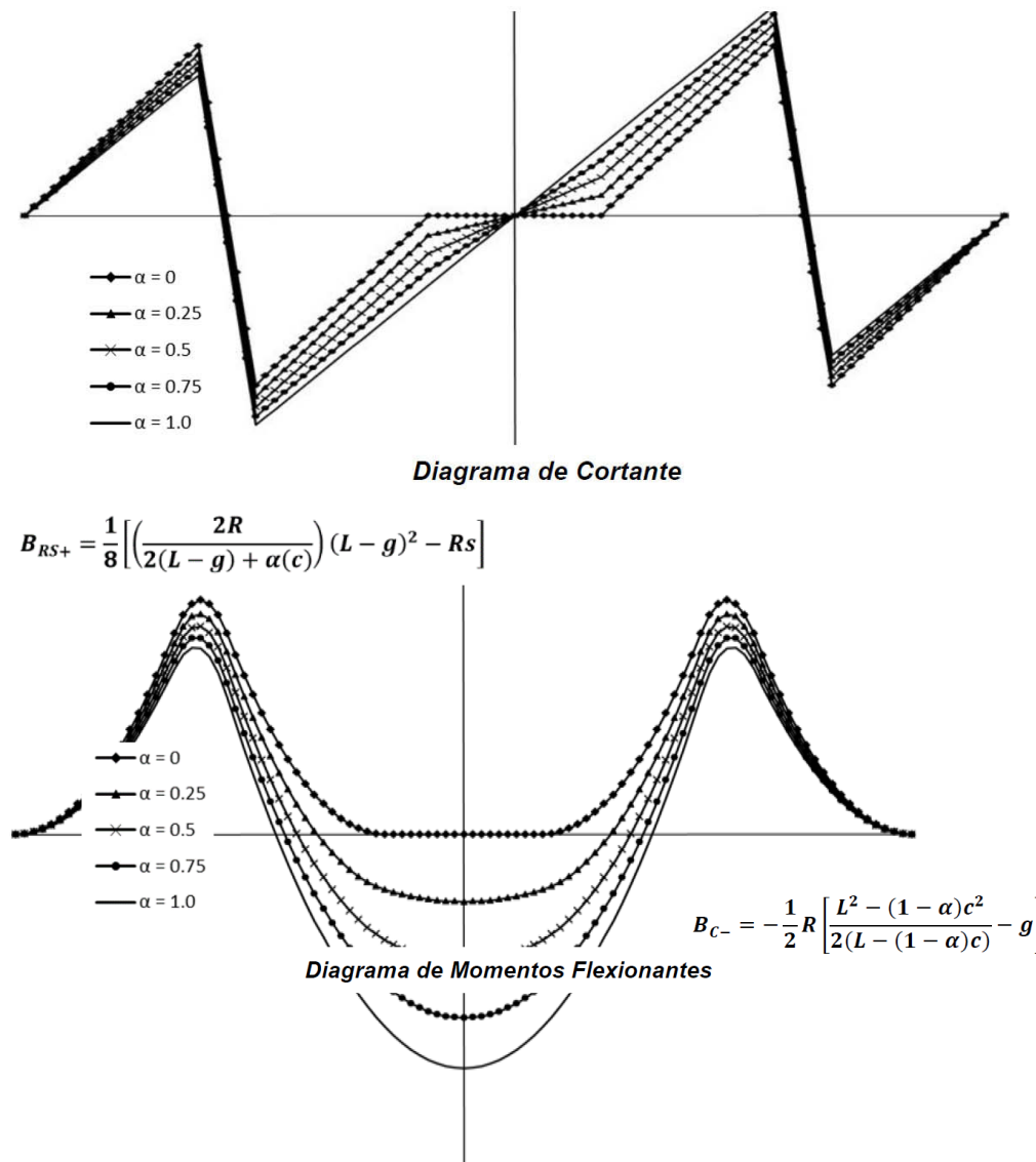
Figura 4. Suposiciones de Carga y Condiciones de Soporte, Diagrama de Cortante y Diagrama de Momento Flexionantes para la Determinación de Momentos Flexionantes de Diseño
