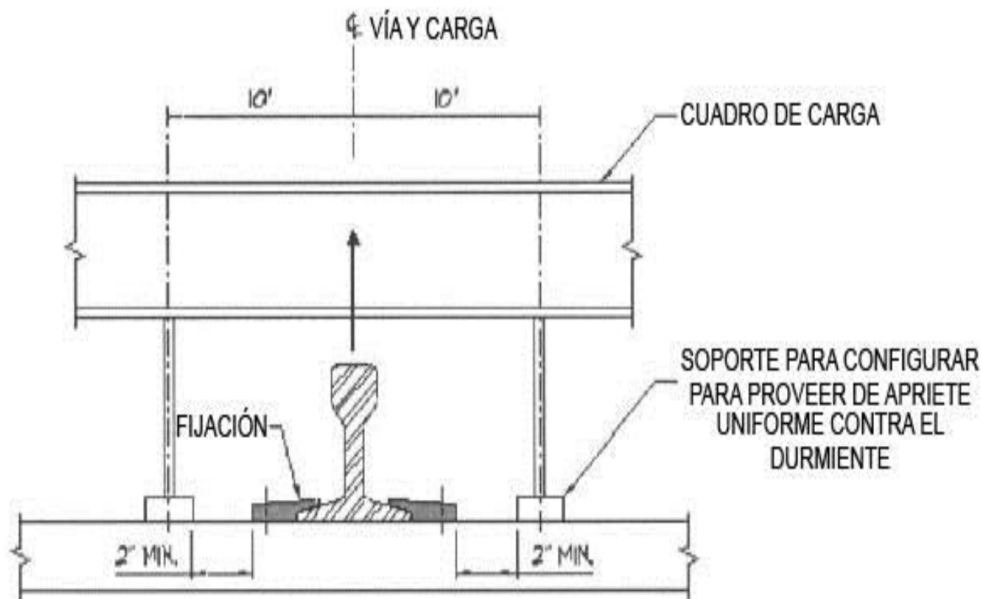
Figura 14. Prueba de extracción de Fijación
