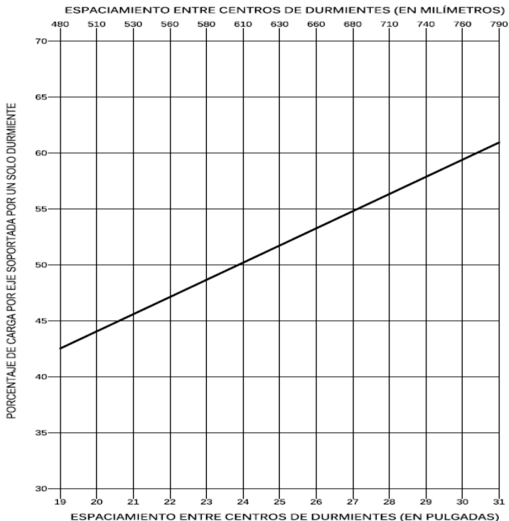
Figura 1. Distribución de carga Estimada
