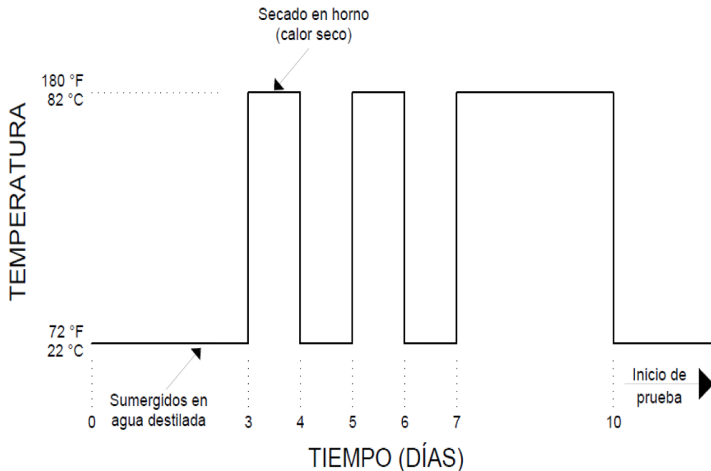
Figura 7. Ciclo de tratamiento
