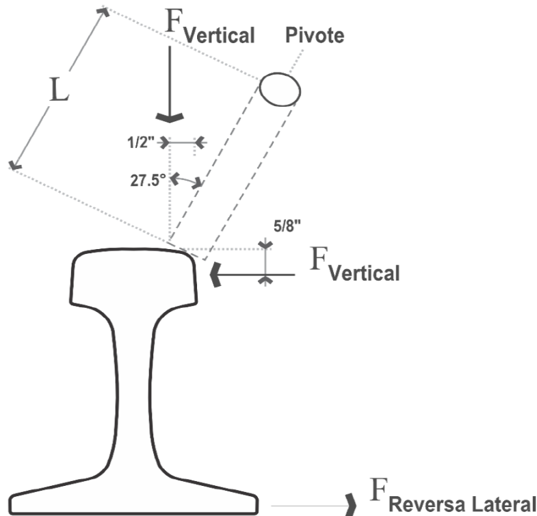
Figura 17. Diagrama de cargas
