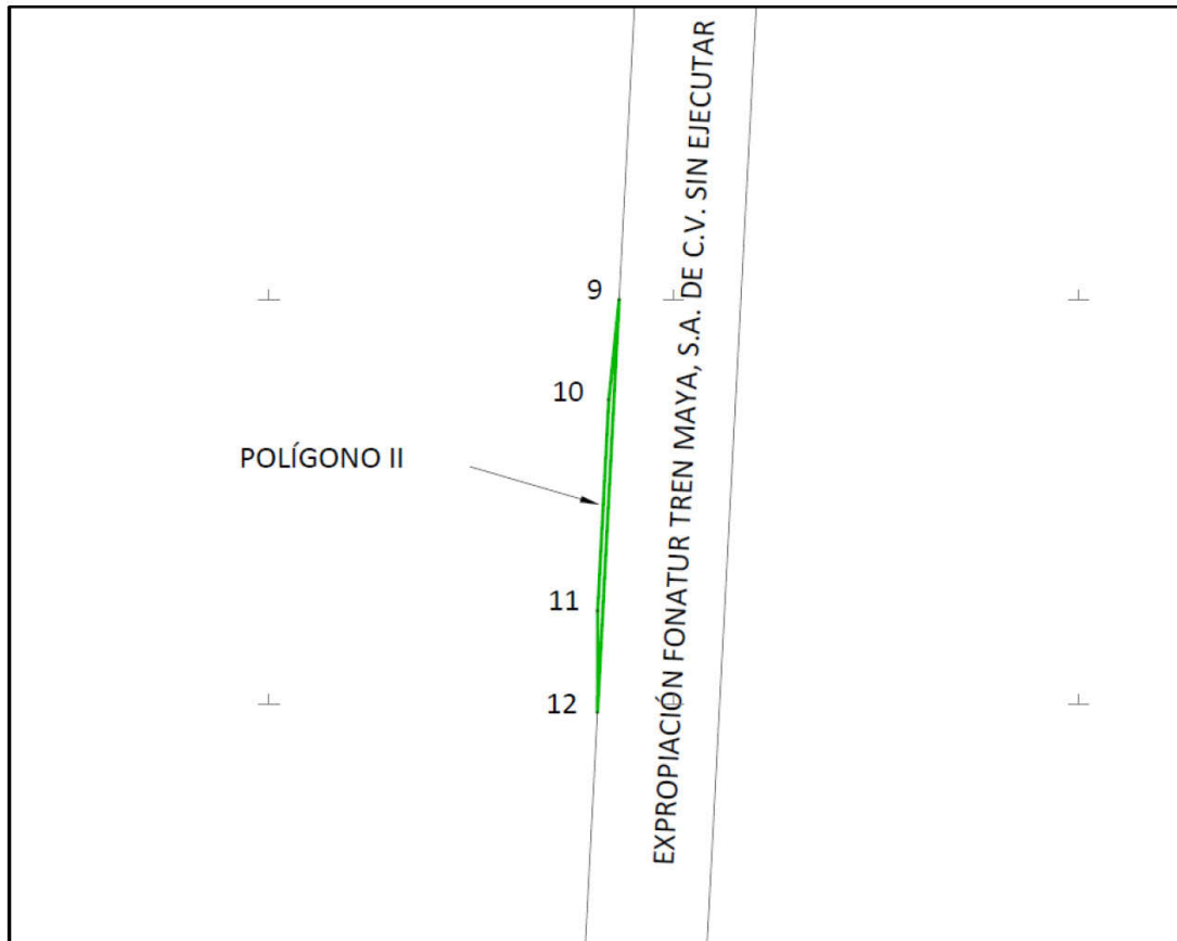
CUADRO DE CONSTRUCCIÓN POLÍGONO II, AFECTACIÓN A TIERRAS DE USO COMÚN ZONA 1
