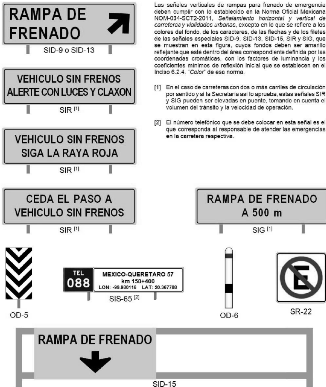
Figura 8.- Señales verticales de rampas para frenado de emergencia
