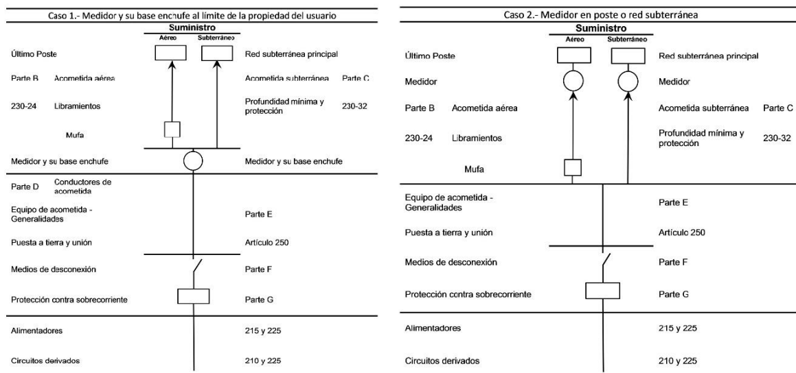
Figura 230-1.- Acometidas
