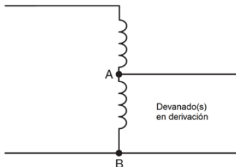
Figura 450-4.- Autotransformador
