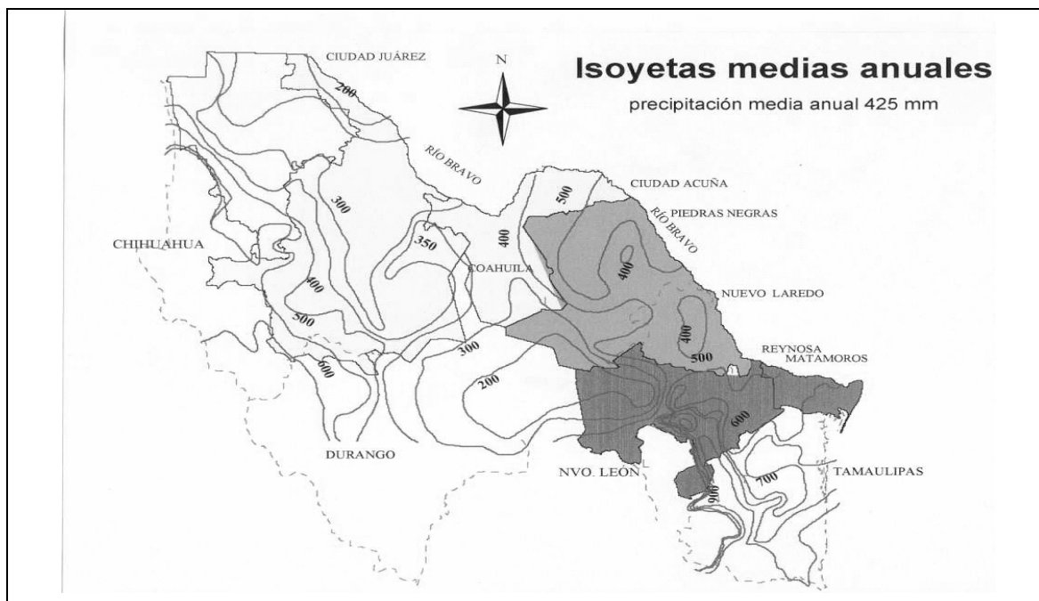
Figura 7.- Mapa de isoyetas medias anuales en la Región Hidrológica número 24 Bravo-Conchos
