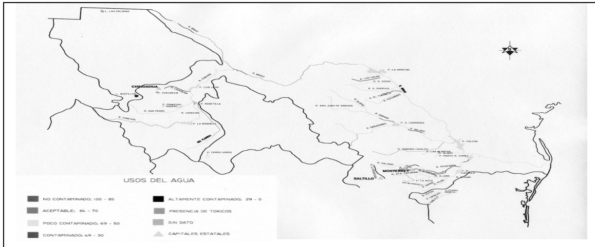
Figura 10.- Mapa de Calidad del Agua superficial en el Río Bravo y sus principales afluentes
