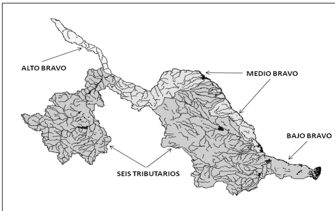
Figura 5.- Subregiones Hidrológicas de la Región Hidrológica número 24 Bravo-Conchos
