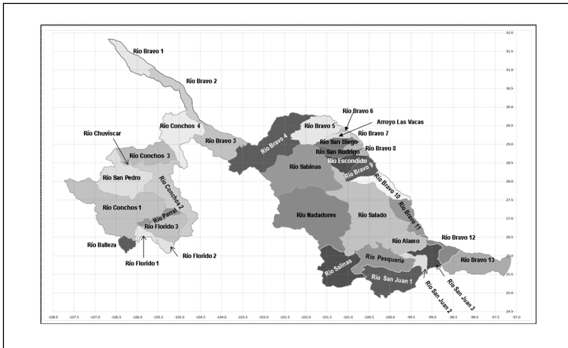
Figura 4.- Cuencas Hidrológicas de la Región Hidrológica número 24 Bravo-Conchos
