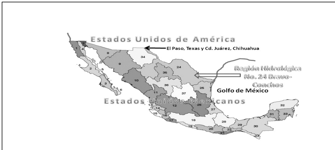
Figura 1.- Región Hidrológica número 24 Bravo-Conchos.
