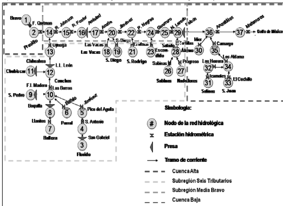
Figura 9. Diagrama unifilar de la Región Hidrológica número 24 Bravo-Conchos para cálculo de disponibilidad
