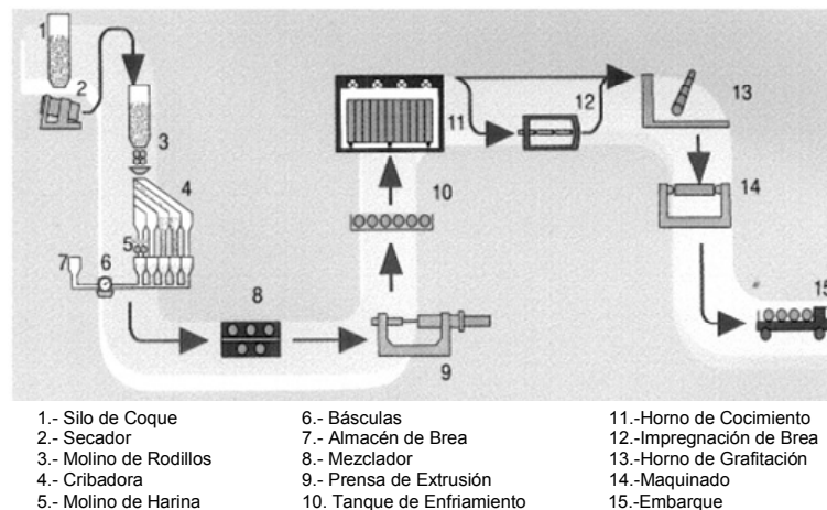
Diagrama 1. Flujo de la producción de electrodos de grafito
